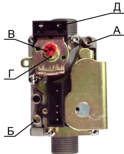
Рис. 7 Регулятор подачи газа
